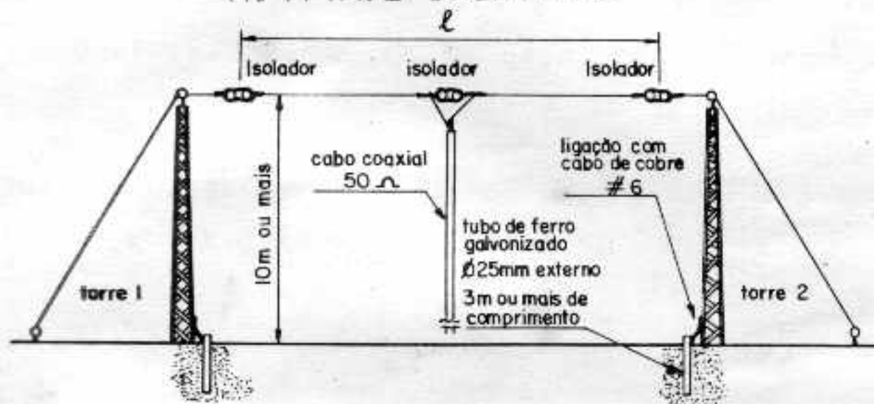
Fig 14 AWG ENLAPADO
